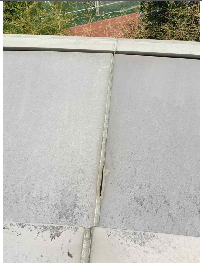
외부 판넬 틈새(누수 원인 추정)
