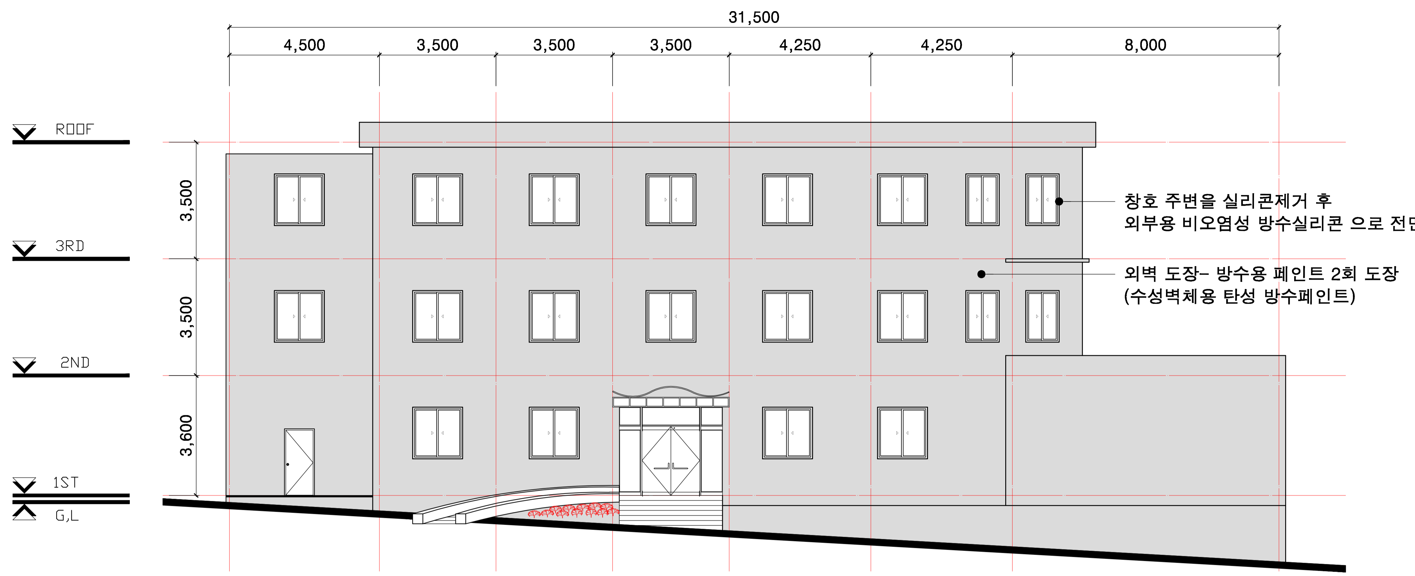
정면도 (SCALE 1/150)
