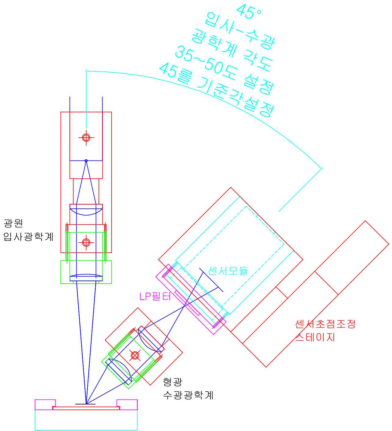
광학계 설계 정면도 (챔버 정면에서 본 구조도)
