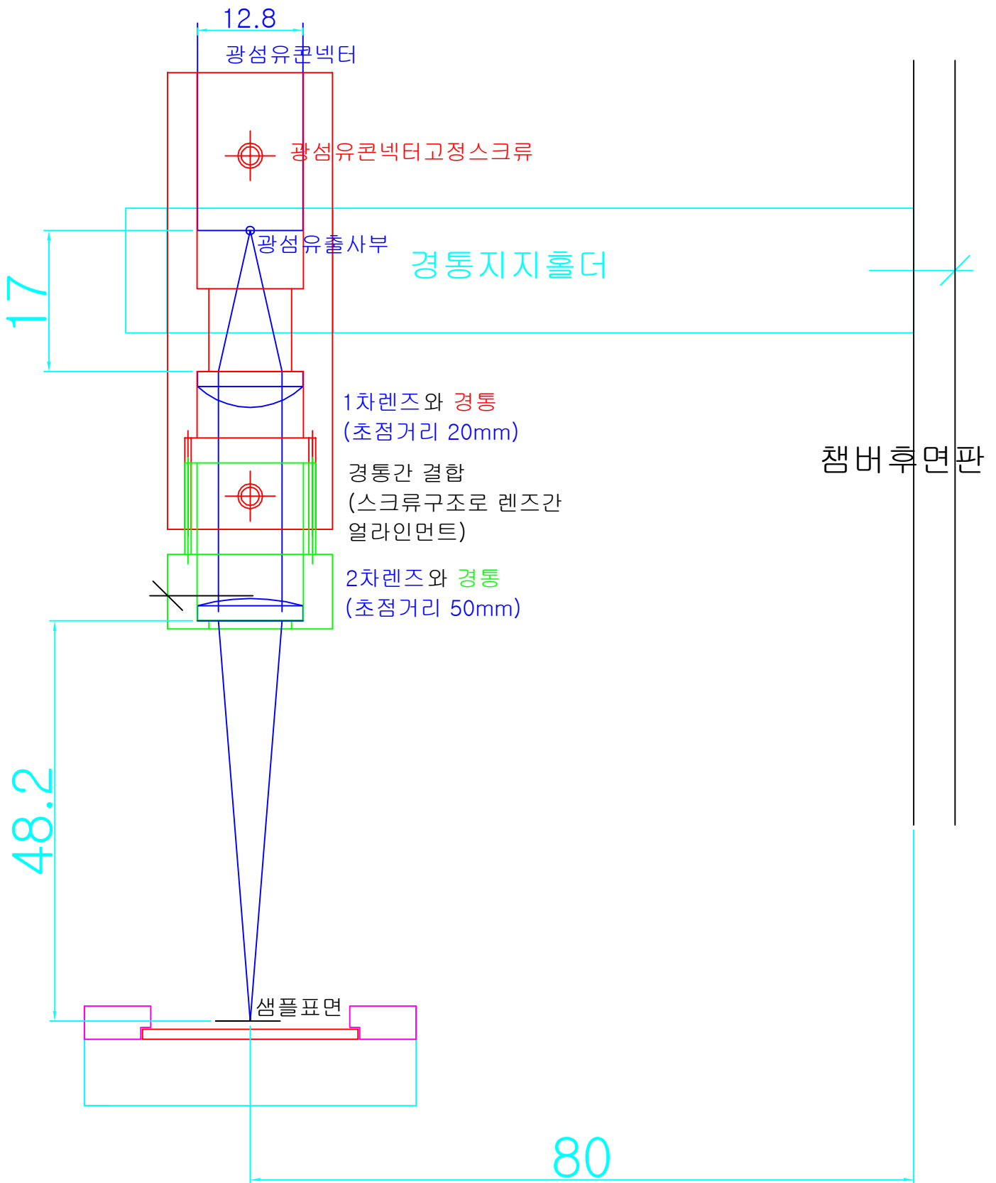
광원입사광학계 측면도 (챔버 우측에서 본 구조도)
