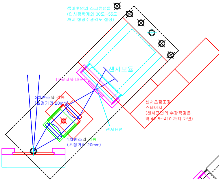
수광광학계와 센서모듈 정면도 (챔버 정면에서 본 구조도)
