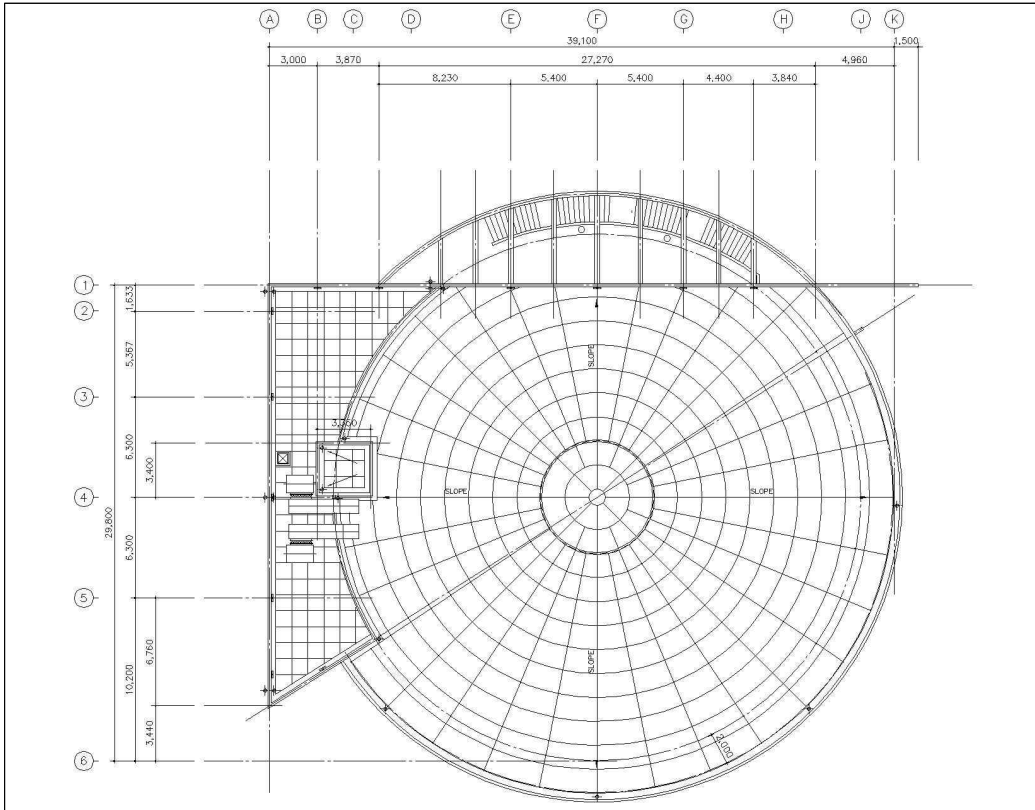
상록원 평면도
