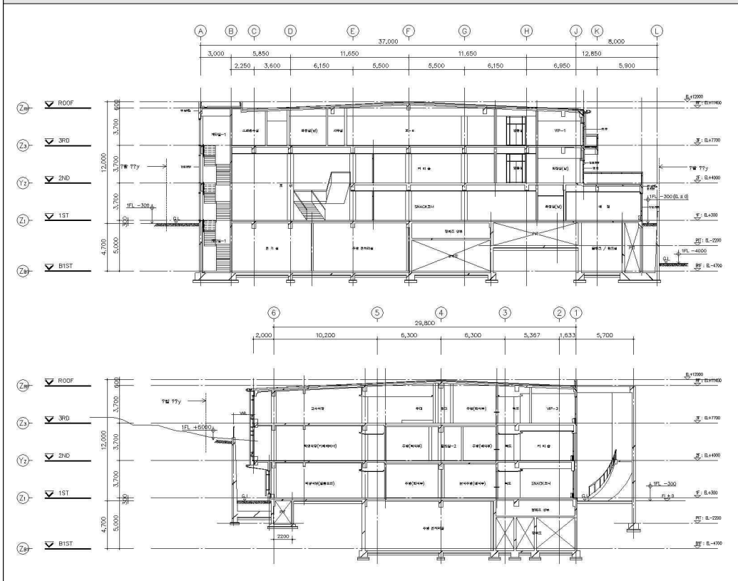
상록원 단면도
