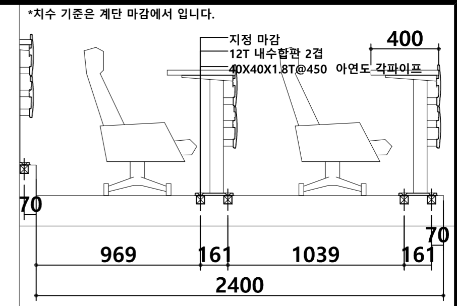
"SK-150-4(TA) 양카 위치 DETAIL"
