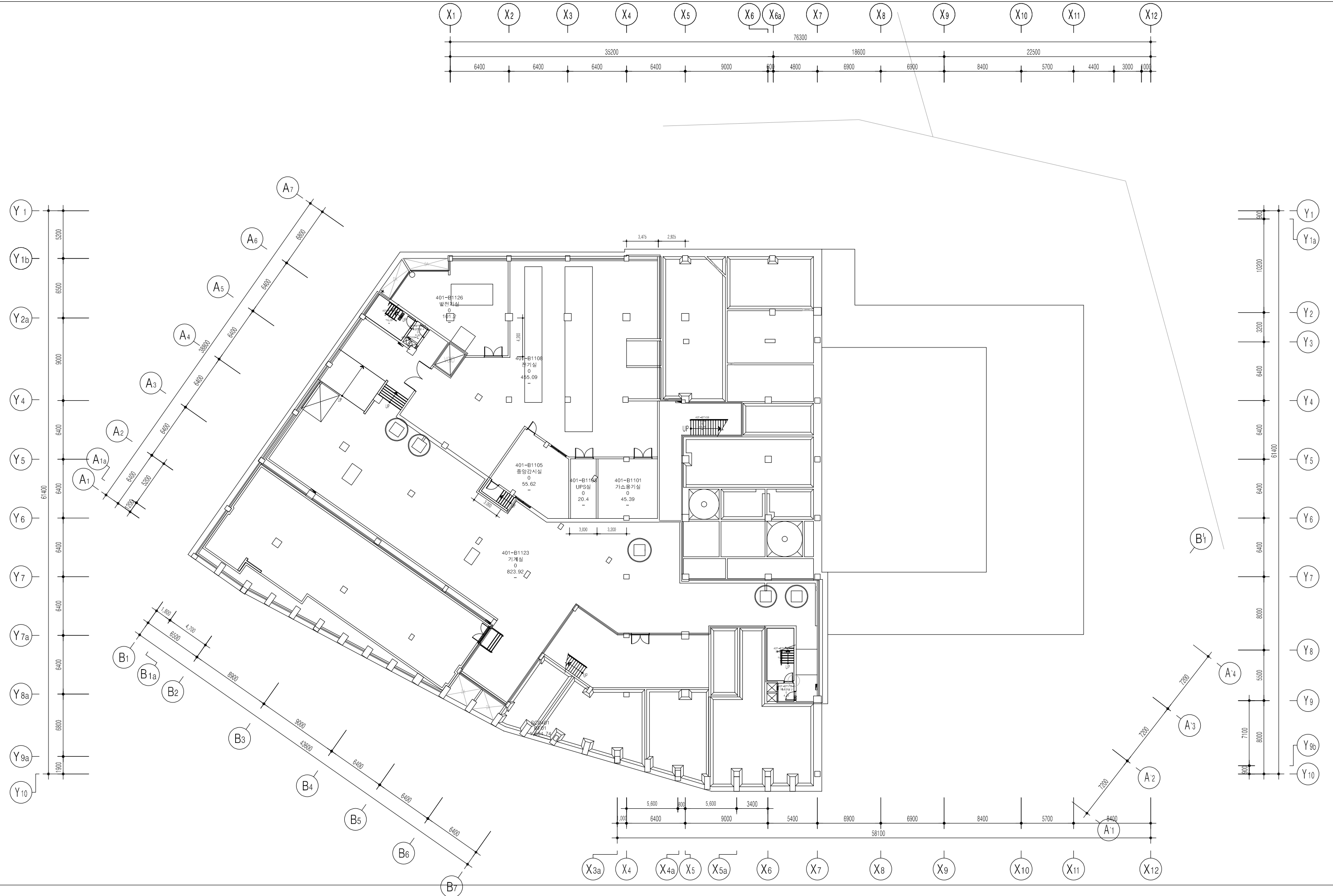
지하 1층 평면도 축척 : 1/400
