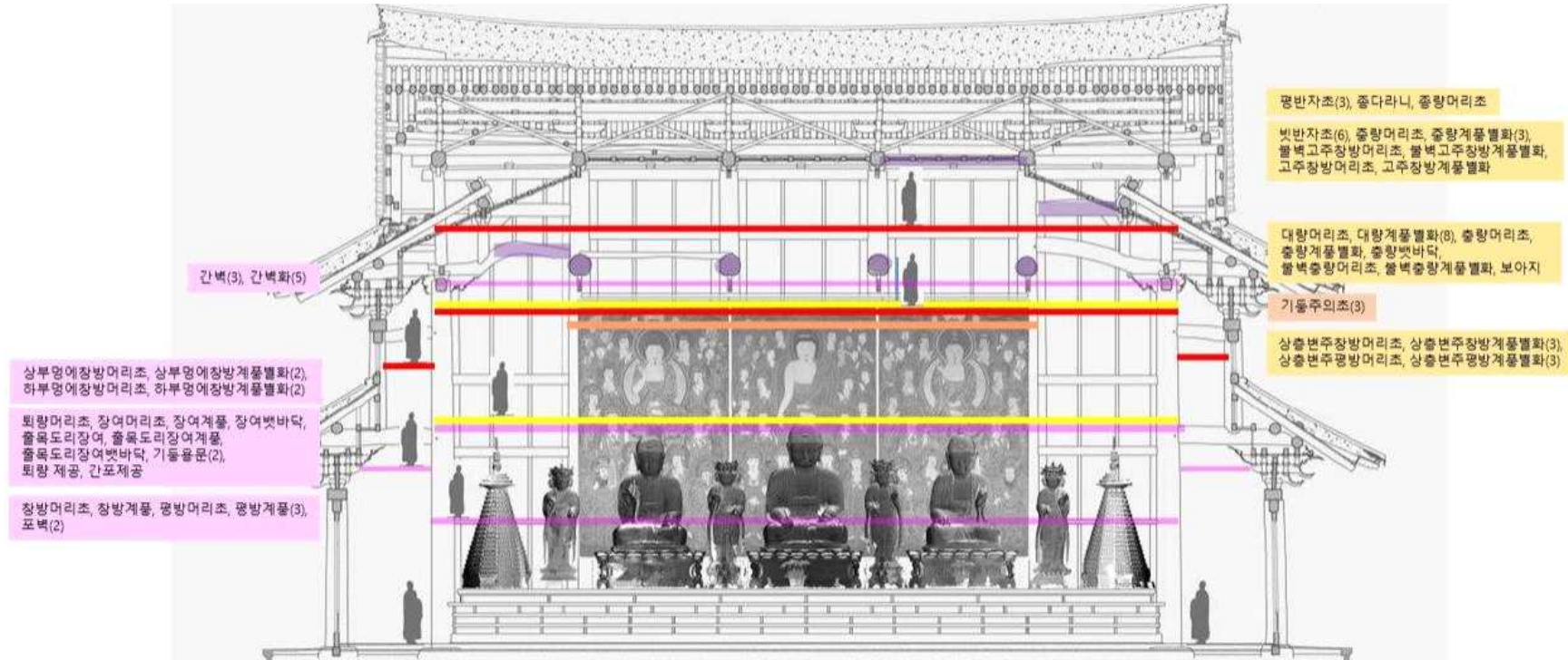
화엄사 각황전 내부 비계 설치 도면(정면)
