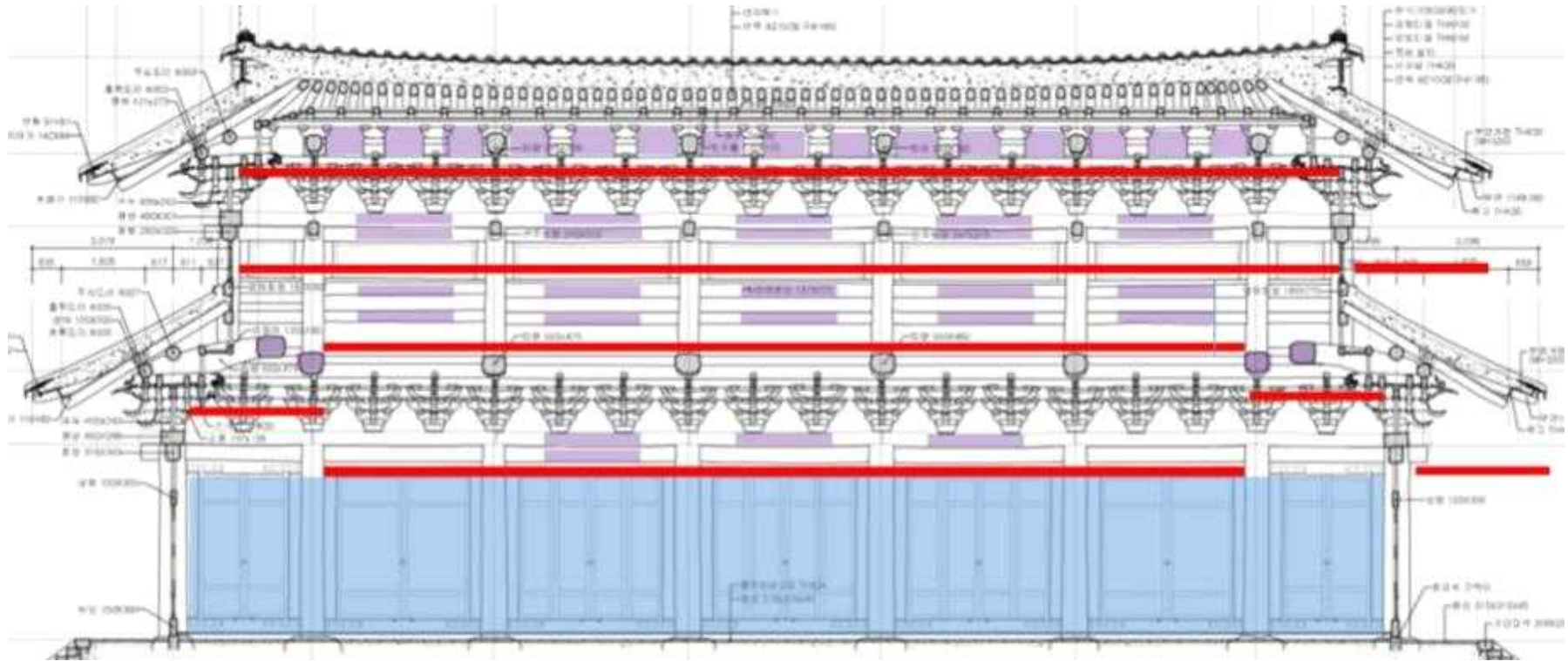
화엄사 각황전 내부 비계 설치 도면(정면)
