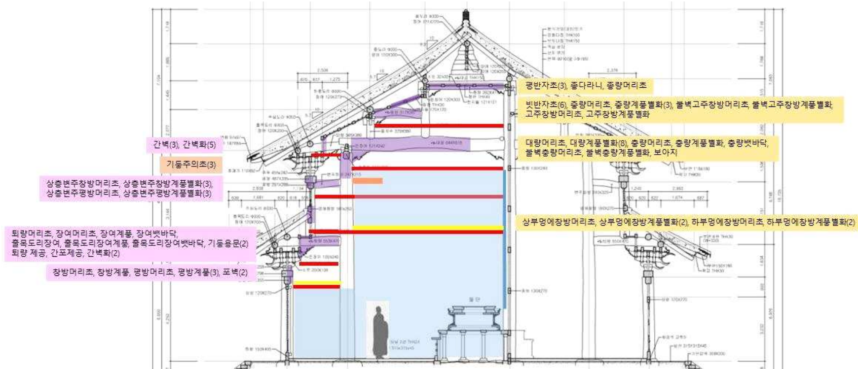
화엄사 각황전 내부 비계 설치 도면(우측면)
